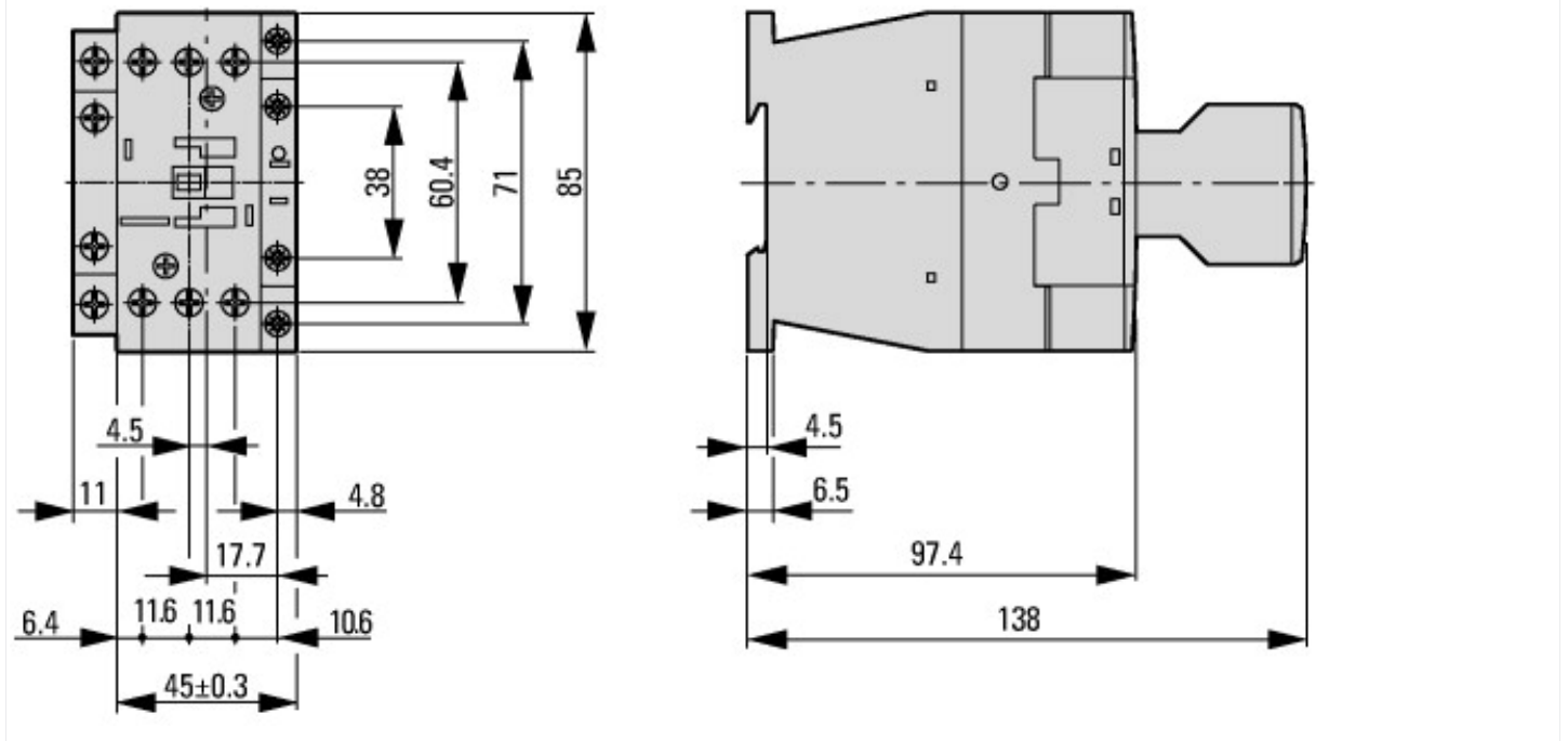
Contacteur with auxiliary contact module
