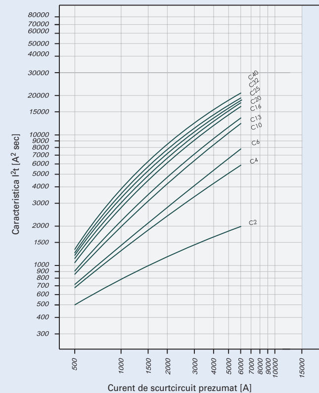
Caracteristica I 2 t maximală pentru PLN6, caracteristică C
