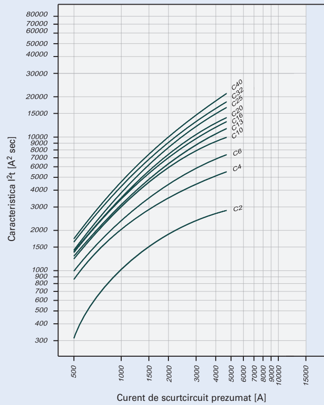
Caracteristica I^2t pentru CKN4, caracteristica C, 1+N-poli
