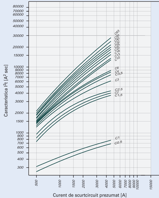
Caracteristica I 2 t pentru CLS4, caracteristică C, 1-poli
