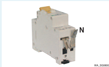
Acelasi unghi de conectare ZV-N-05TE (-80A) pentru baretele N 50 si 80 A
