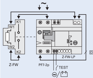
Schema de conexiuni: PF7-2p, alimentare întreruptor diferențial sus
