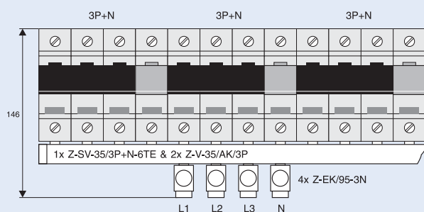
Secțiunea conductorului de racordare 25 - 95 mm 2
