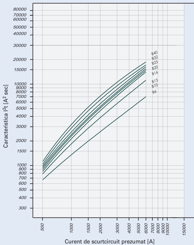
Caracteristica I 2 t maximală pentru PLN6, caracteristică B
