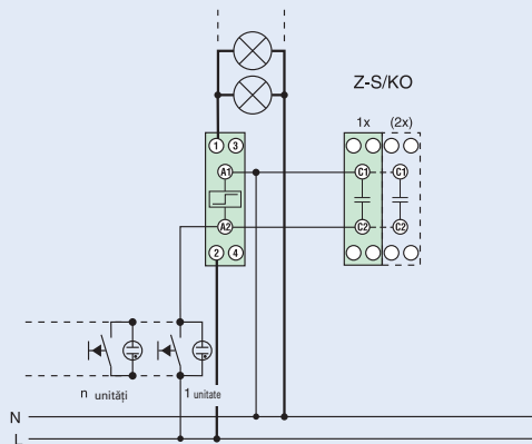
Compensare cu bloc condensatoare
