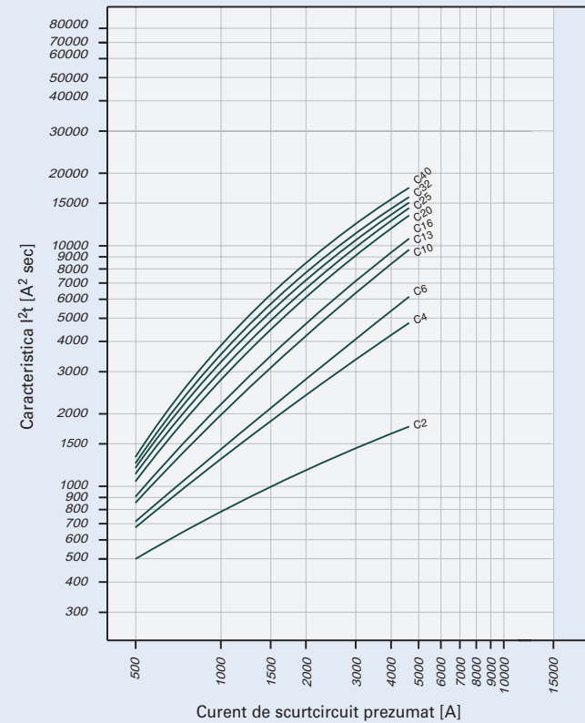
Caracteristica I 2 t maximală pentru PLN4, caracteristică C
