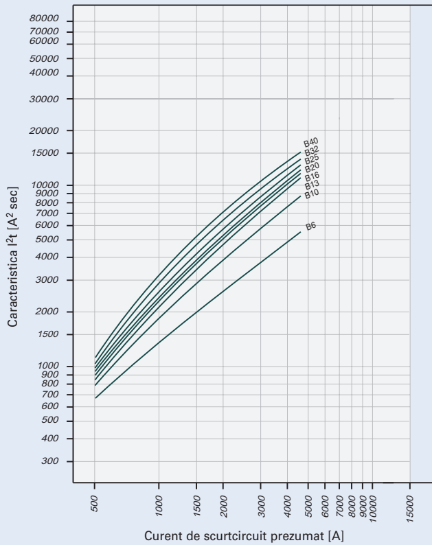
Caracteristica I 2 t maximală pentru PLN4, caracteristică B
